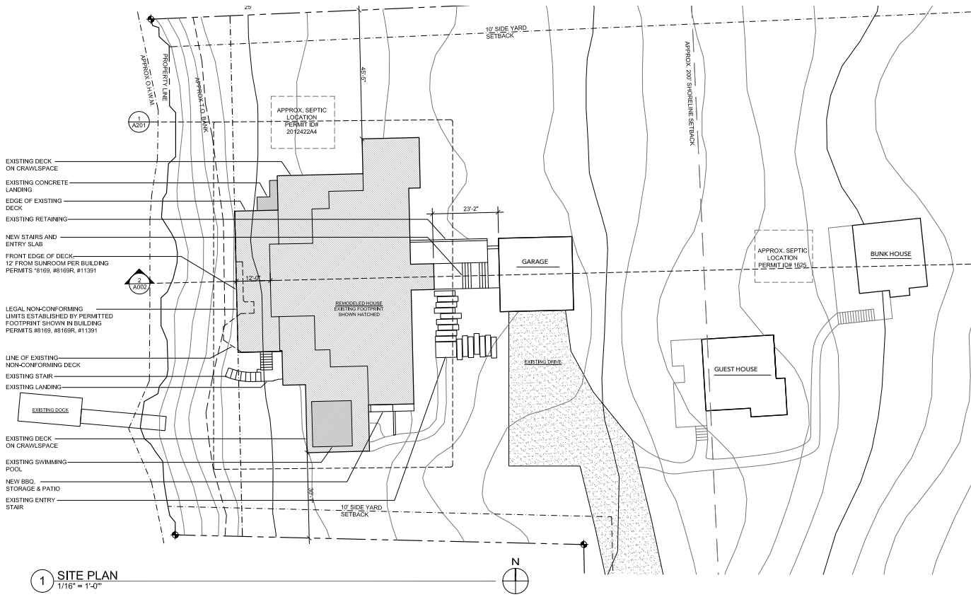
3 POLARIS SITE PLAN
